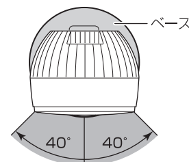
首振り範囲：80°
